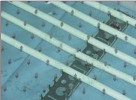
Рис. 11.13. Укладка трубы «теплого пола» в краевой зоне
