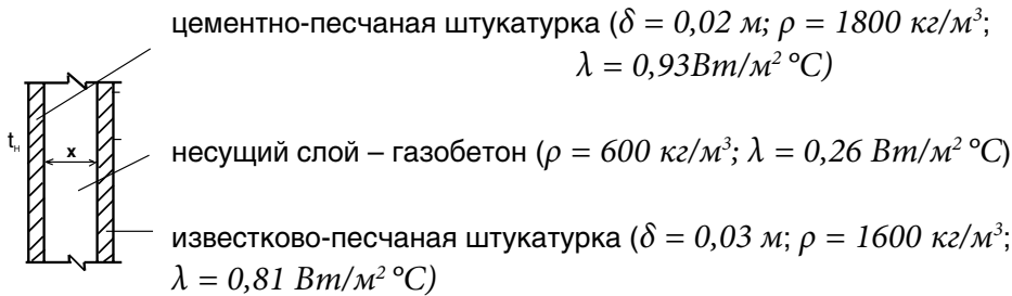
Рис. 7.4. Наружная стена
