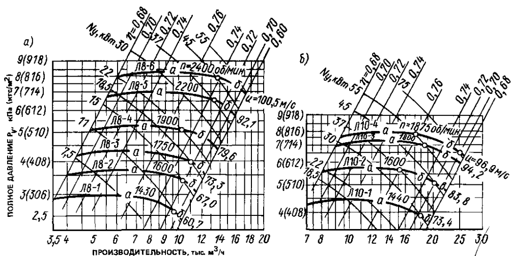
Рис. 1.21. Аэродинамические характеристики вентиляторов В.Ц6-28-8 (а) и В.Ц6-28-10 (б) (исполнение 6)
