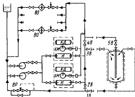
Рис. 16.9. Схема закрытой системы циркуляции холодоносителя с вертикальным баком-аккумулятором
