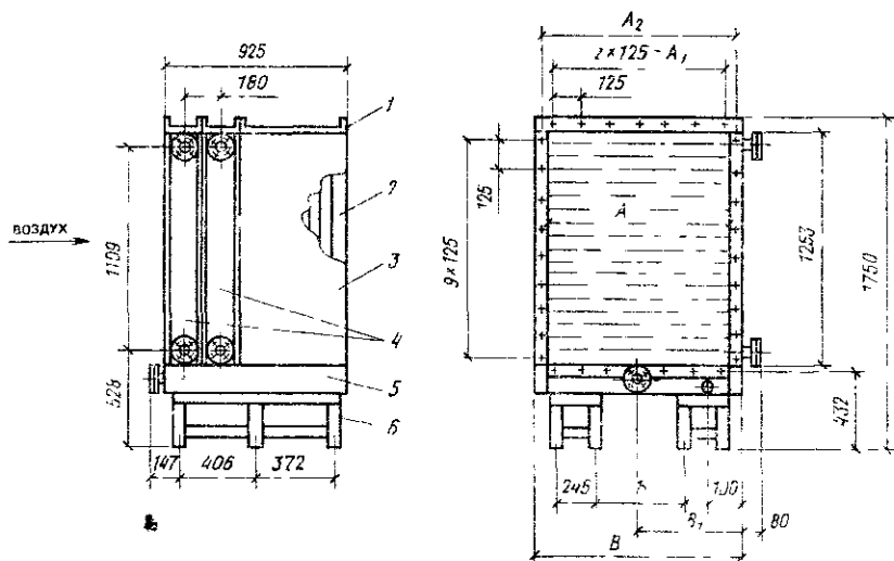
Рис III 7 Блоки теплоутилизации БТ-3
