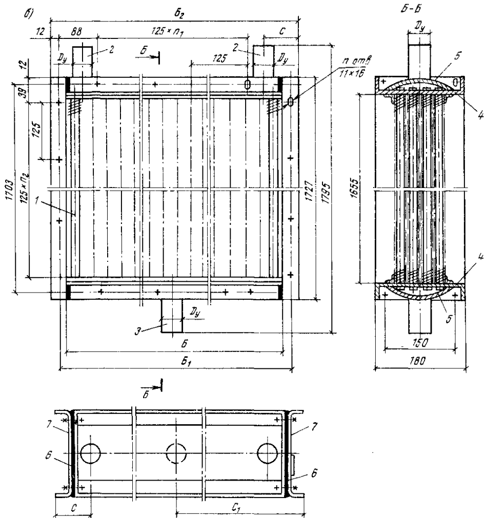
Рис. II.3. Воздухонагреватели (калориферы) КП36-СК-01УЗА – КП310-СК-01УЗА(а), КП311-СК-01УЗА и КП312-СК-01УЗА (б)
