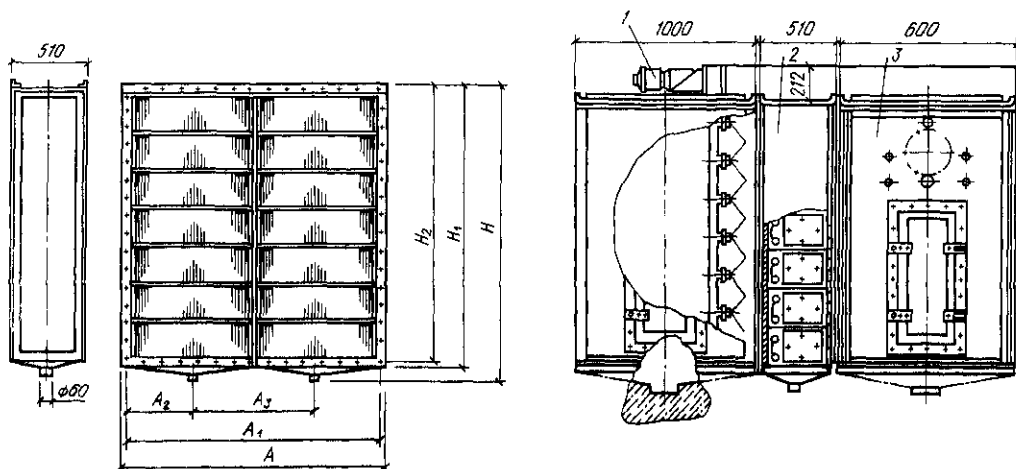
Рис. IV.5. Электрофильтр ФЭ
