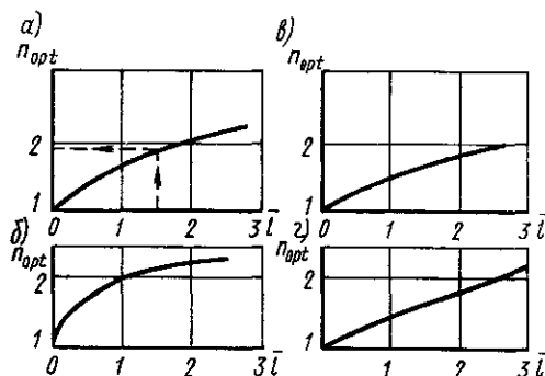
Рис. 22.4. Оптимальные геометрические характеристики конических диффузоров, размещенных на выходе радиальных вентиляторов с лопатками, загнутыми вперед (а), и с лопатками, загнутыми назад (б), плоских диффузоров, размещенных на выходе радиальных вентиляторов с лопатками, загнутыми вперед (в), и с лопатками, загнутыми назад (г)
