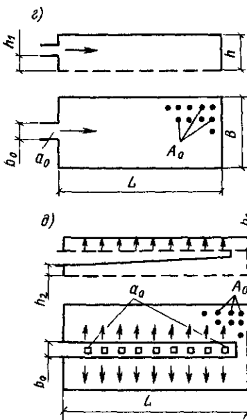
Рис. 17.8. Схемы подачи воздуха в подшивное пространство
