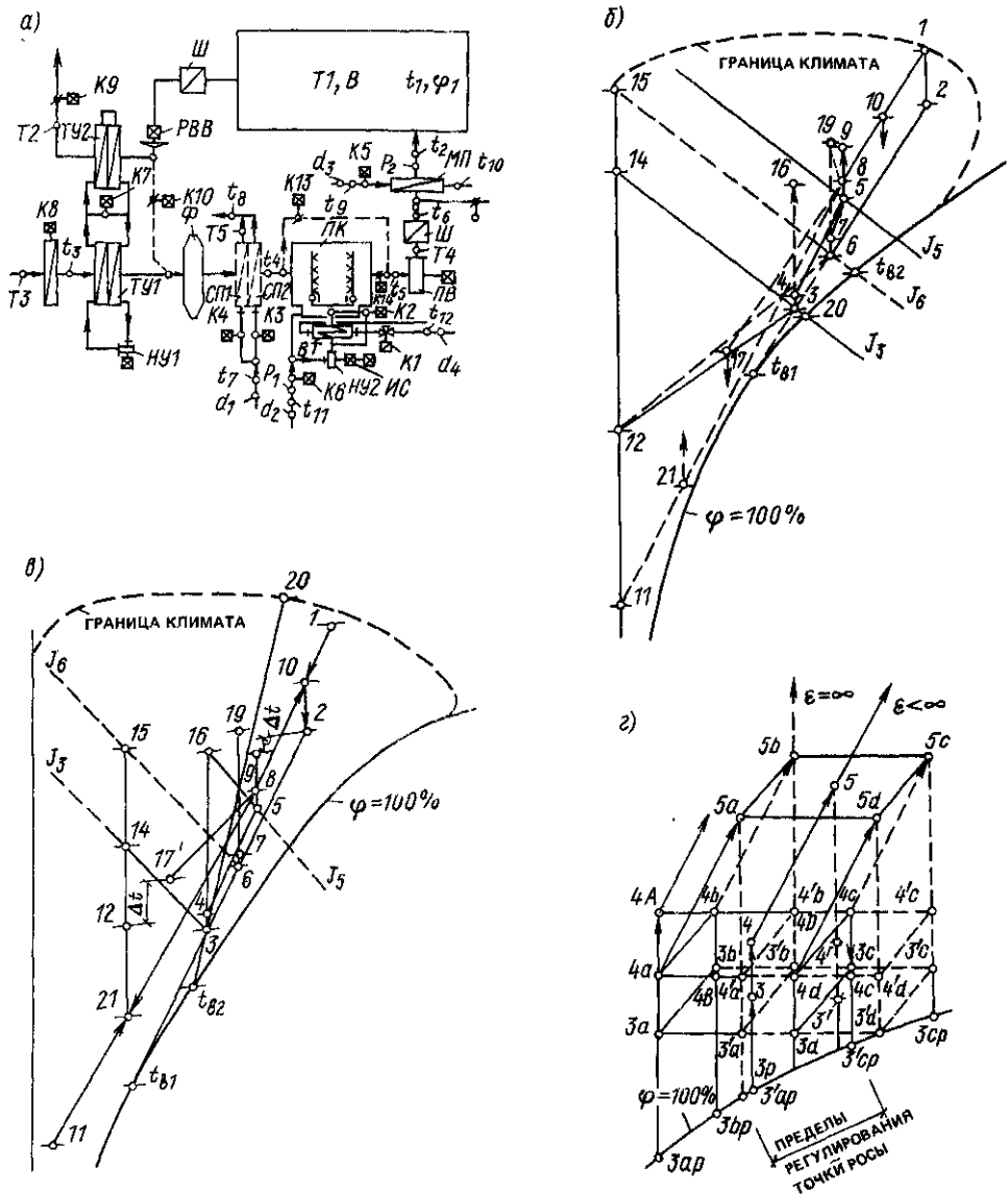
Рис. 15.8. Центральная приточная однозональная система кондиционирования воздуха, работающая полностью на наружном воздухе или с рециркуляцией (рециркуляционный воздуховод и клапан К10 показаны пунктиром)
