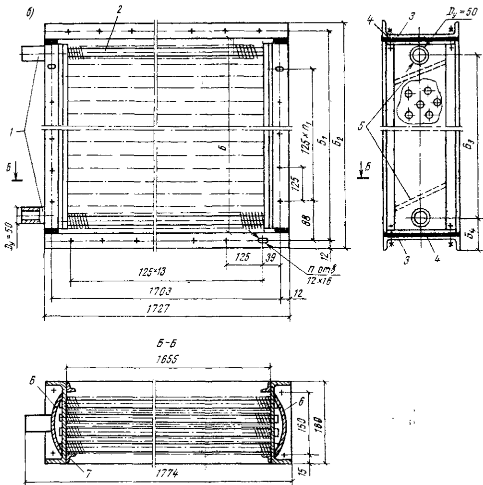
Рис. П.2. Калориферы КСК4-6-02ХЛЗА – КСК4-10-02ХЛЗА (а) и КСК4-11-02ХЛЗА и КСК4-12ХЛЗА (б) 1 патрубki для подвода и отвода теплоносителя; 2 – теплопередающая трубка теплообменного элемента; 3 – боковые щитки; 4 – уплотнительные прокладки; 5 – перегородки в распределительно-сборных коллекторах; 6 – крышка; 7 – грубая решетка
