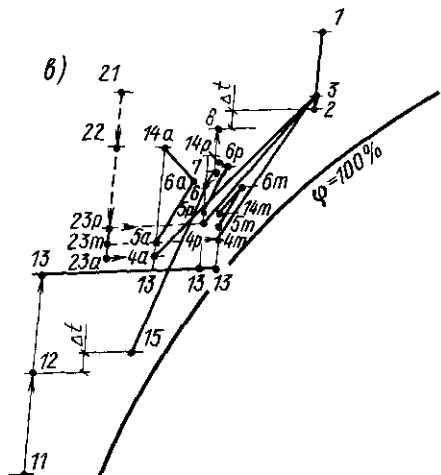
Рис. 15.13. Центральная многозональная система кондиционирования воздуха с увлажнением воздуха паром
