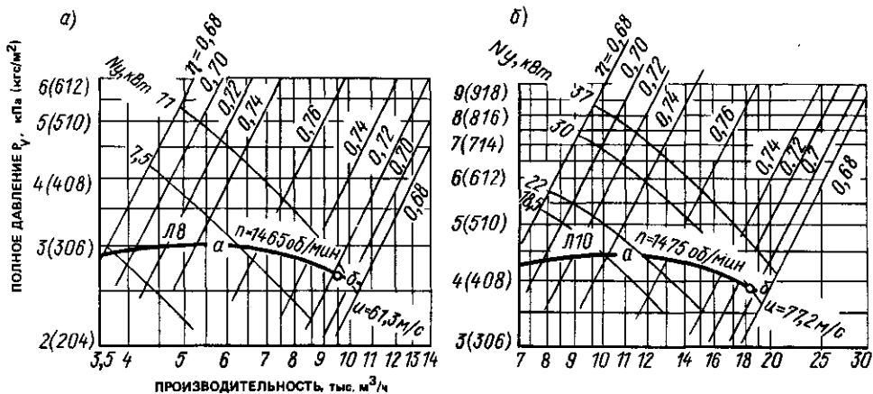
Рис. 1.20. Аэродинамические характеристики вентиляторов В.Ц6-28-8 (а) и В.Ц6-28-10 (б) (исполнение 1)
