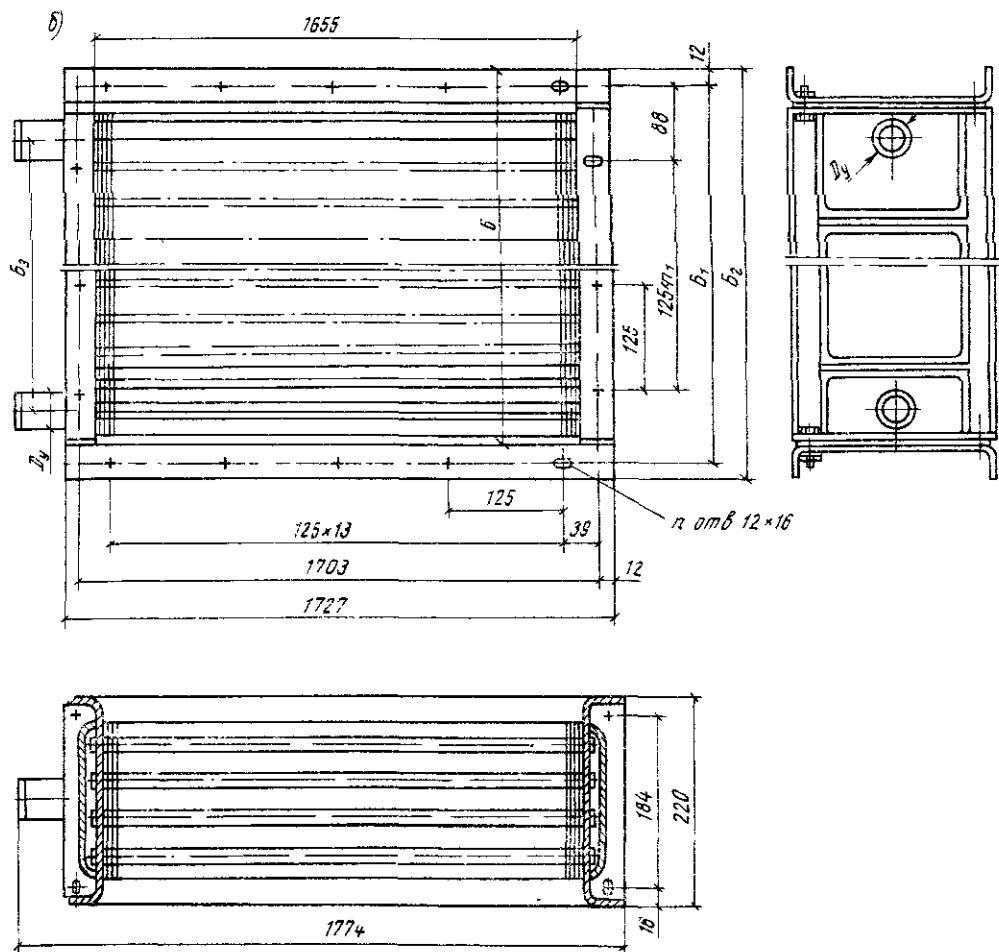
Рис. II.7. Калориферы стальные пластинчатые КВБ6Б – КВБ10Б (а), КВБ11Б и КВБ12Б (б)
