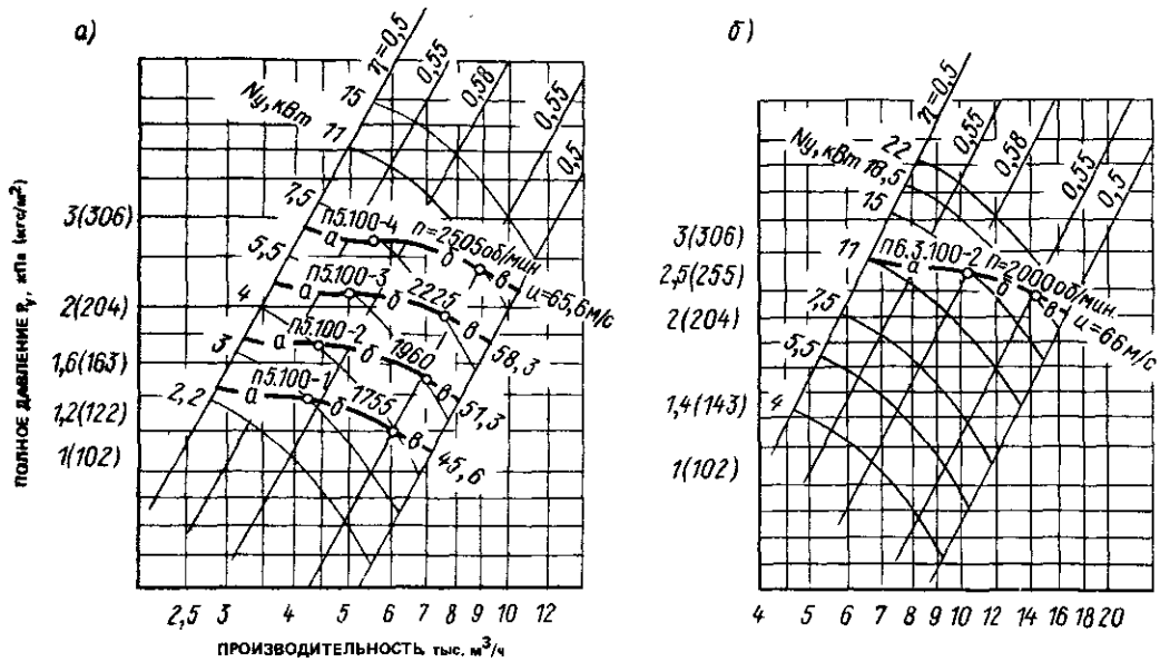
Рис. 1.23. Аэродинамические характеристики пылевых вентиляторов В.ЦП6-45-5 (а) и В.ЦП6-45-6,3 (исполнение б)
