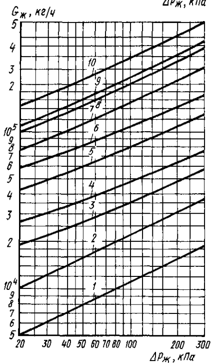
Рис 15.32 Зависимость давления воды перед форсунками \Delta P_{ж} от расхода воды G_{ж} для двухрядных камер орошения ОКФ-3
