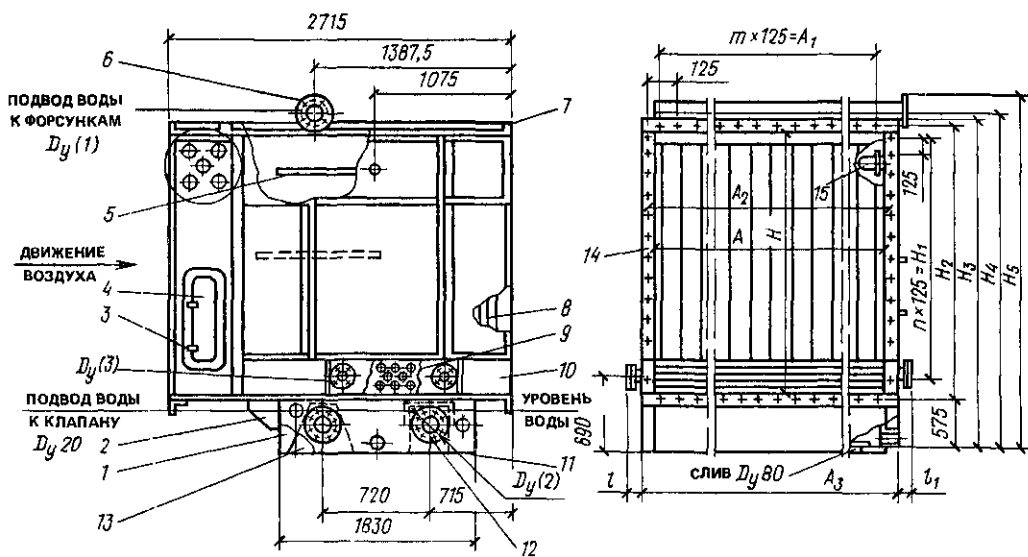
Рис III 4 Камеры орошения ОКС2-3 (КТЦ3-31,5, КТЦ3-40, КТЦ3-63, КТЦ3-80)
