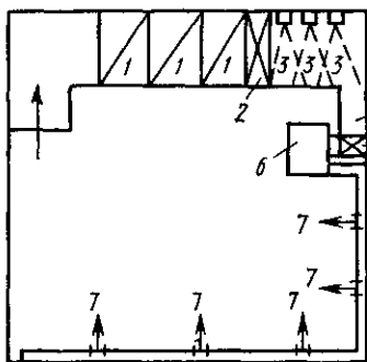
Рис. 15.61. СКВ с установкой для дезодорации воздуха
