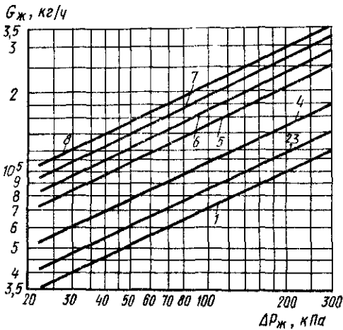
Рис. 15.35. Зависимость давления воды перед форсунками \Delta P_{ж} от расхода воды G_{ж} для камер орошения ОКС-3
