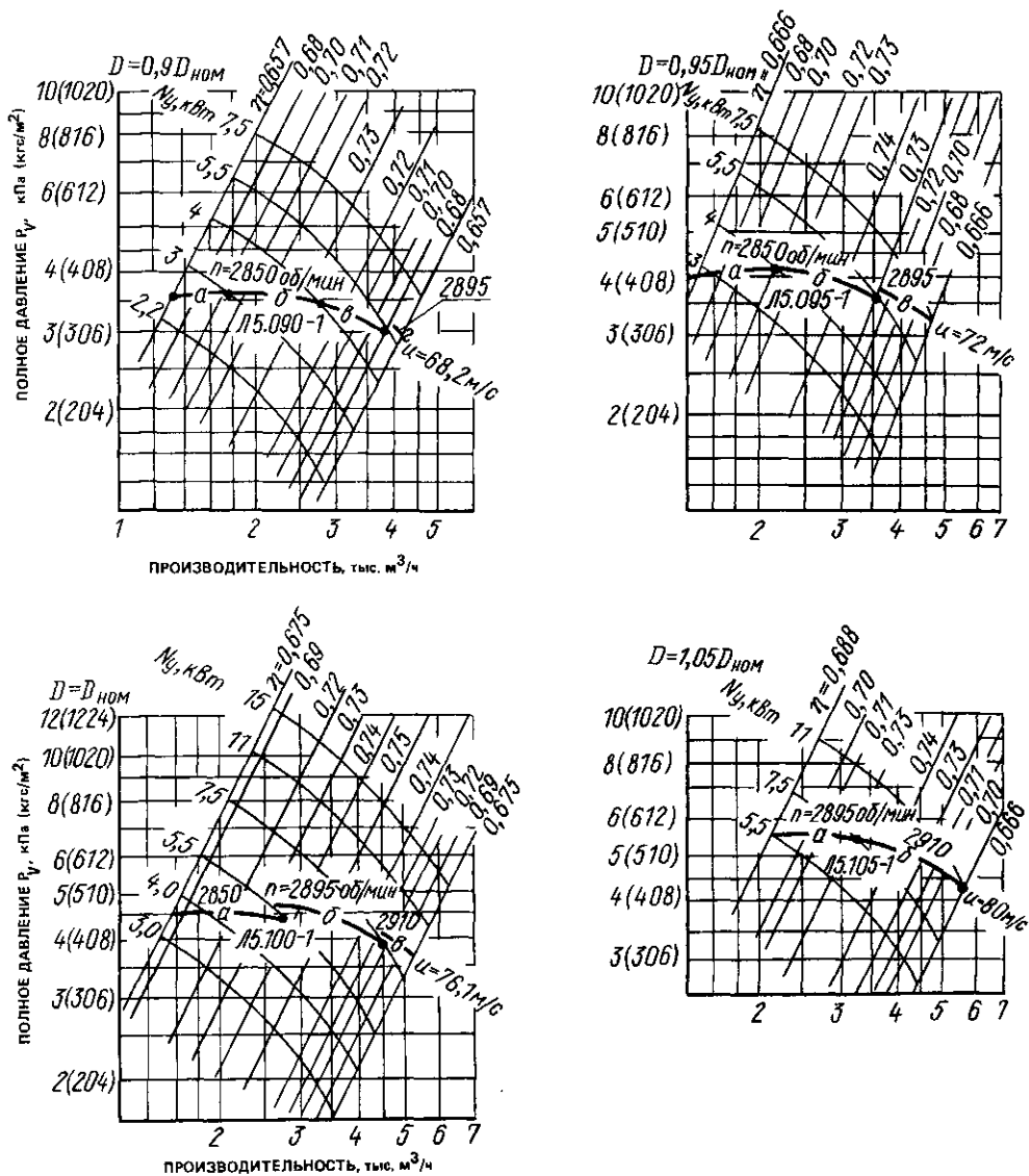
Рис. 1.18. Аэродинамические характеристики вентиляторов В.Ц6-28-5 (исполнение 1)
