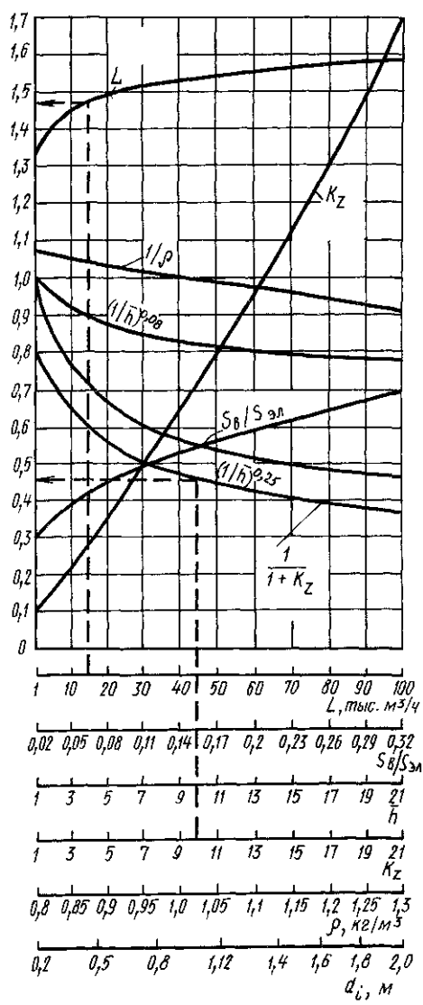
Рис. 22.2. Номограмма вспомогательных величин для определения v^*
