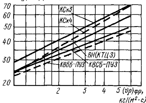
Рис. 21.11. Определение коэффициентов наружного теплообмена для воздухонагревателей типа КСк3, КСк4, КВСБ-ПУЗ, КВББ-ПУЗ и ВН
