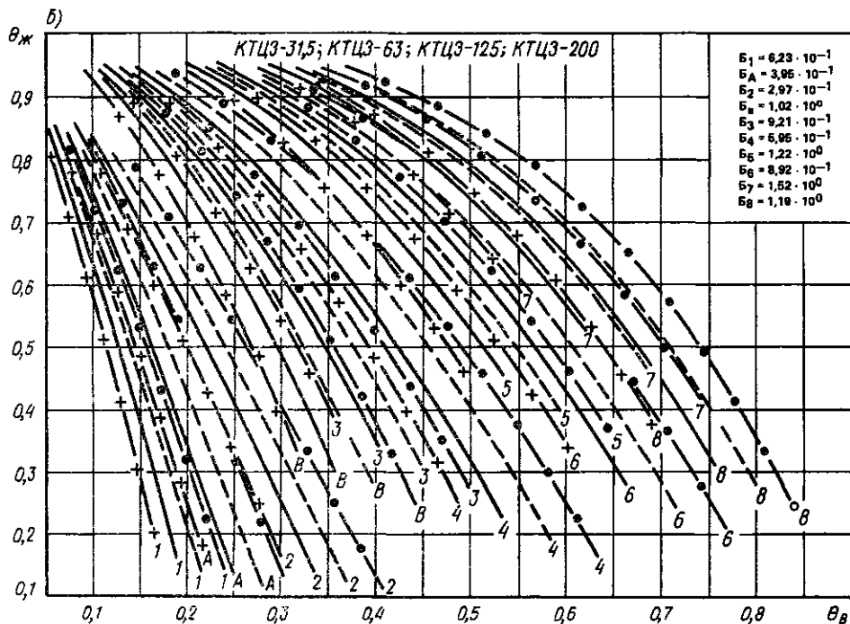
Рис. 15.41. Теплоэнергетические и гидравлические характеристики теплообменников кондиционеров КТЦЗ-31,5; КТЦЗ-40; КТЦЗ-63; КТЦЗ-80; КТЦЗ-125; КТЦЗ-200 с параллельной схемой обвязки (а, в) и последовательно-противоточной (б, г)
