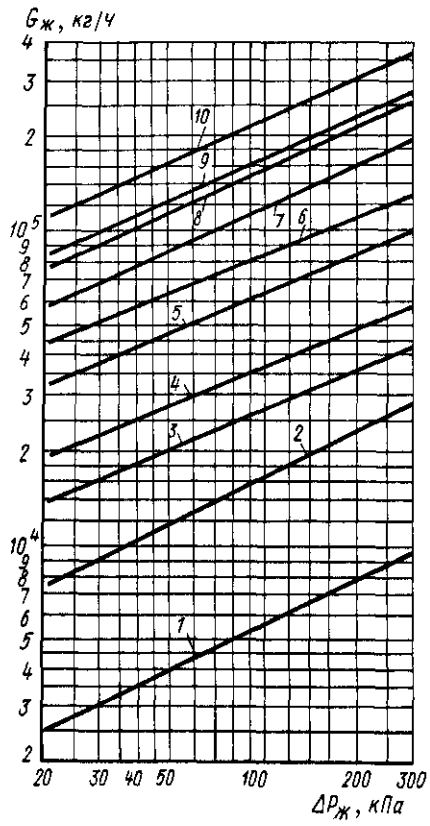
Рис 15.32 Зависимость давления воды перед форсунками \Delta P_{ж} от расхода воды G_{ж} для двухрядных камер орошения ОКФ-3
