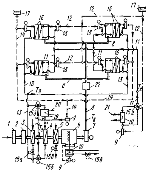
Рис. 15.20. Схема центральной одноканальной четырехтрубной эжекционной СКВ с вводом к ЭКД холодного первичного воздуха, горячей и холодной воды
