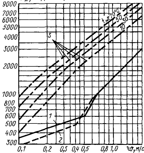
Рис. 21.12. Определение коэффициентов внутреннего теплообмена \alpha_{ж} для воздухонагревателей
