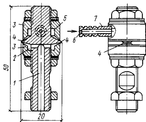
Рис. 15.37 Пневматическая форсунка типа ФД-2 ЦНИИХБ
