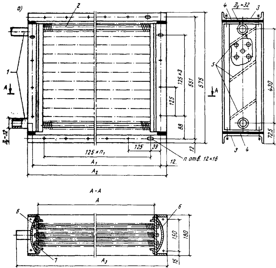
Рис. II.1. Калориферы КСк3-6-02ХЛЗА — КСк3-10-02ХЛЗА (а) и КСк3-11-02ХЛЗА и КСк3-12-02ХЛЗА (б)
