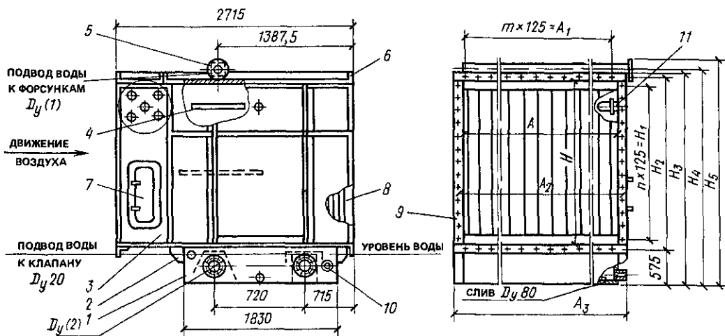
Рис III 3 Камеры орошения ОКС1-3 (КТЦ3-31,5, КТЦ3-40, КТЦ3-63, КТЦ3-80)
