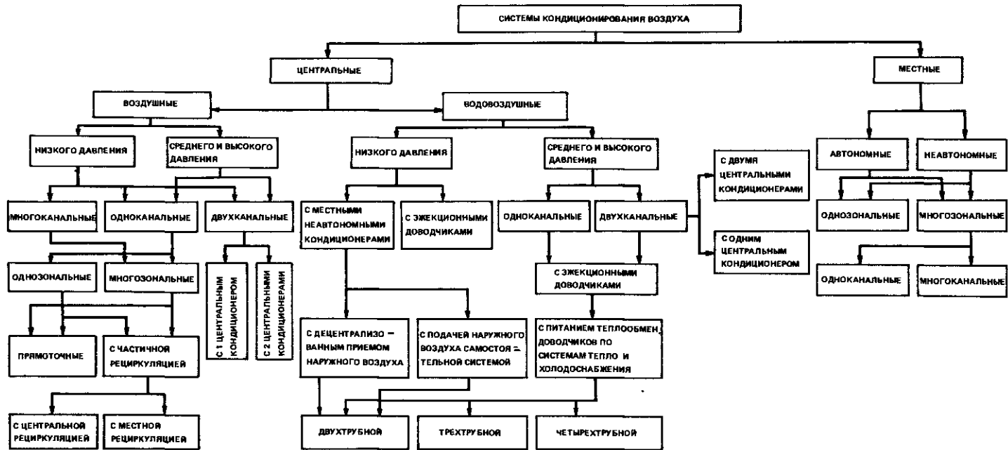
Рис. 15.1. Классификация систем кондиционирования воздуха
