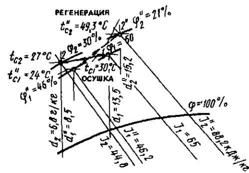
Рис. 15.54. Схема процесса обработки воздуха водным раствором хлористого лития, построенная на t-d -диаграмме
