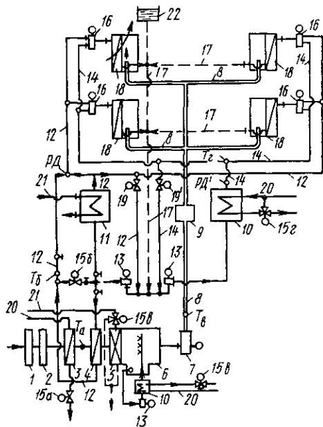
Рис. 15.19. Схема центральной одноканальной трехтрубной эжекционной СКВ с вводом к ЭКД холодного первичного воздуха, горячей и холодной воды.
