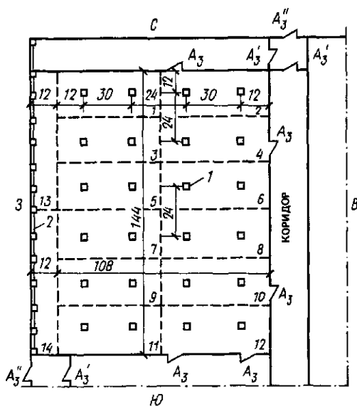
Рис. 20.1. План цеха к примеру расчета 20.1 ( A_3 — эвакуационные выходы из горящего помещения)
