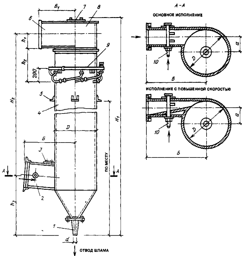
Рис. IV.28. Пылеуловители ЦВП
