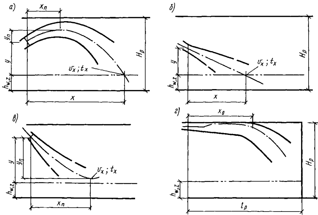
Рис. 17.3. Схемы подачи охлажденного воздуха вверх под углом к горизонтальной плоскости (а), нагретого воздуха вниз под углом к горизонтальной плоскости — ось струи пересекает ПЗ (б) и ось струи выше ПЗ (в), схема настилающей подачи охлажденного воздуха (г)
