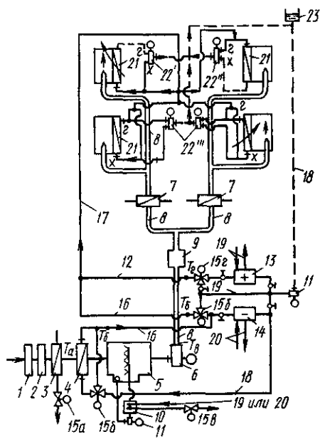
Рис. 15.18. Схема центральной одноканальной двухтрубной эжекционной СКВ с вводом к ЭКД сезонно холодного воздуха и горячей воды или теплого воздуха и холодной воды
