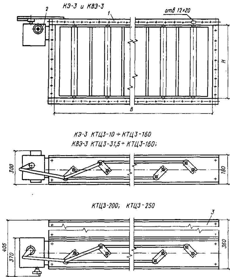
Рис. III.11. Клапаны воздушные КЭ-3 и KBЭ-3
