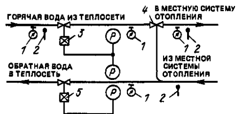
Рис 19.2 Тепловой ввод с элеватором 1 манометр, 2-термометр, 3 регулятор расхода воды в системе отопления, 4 элеватор, 5 регулятор давления (подпора) в обратном трубопроводе системы отопления
