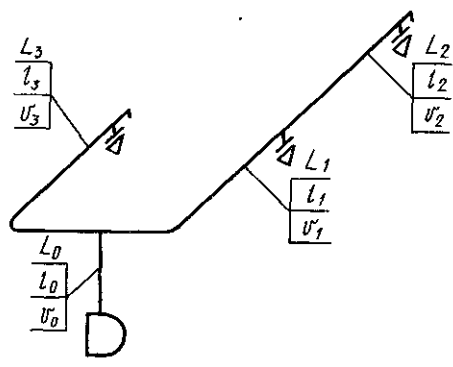
Рис. 22.3. Расчетная схема сети воздухопроводов для определения экономической целесообразной скорости воздуха
