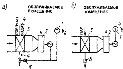
Рис. 19.4. Отопительные агрегаты с теплоносителем водой (а) и теплоносителем паром (б)
