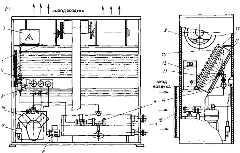
Рис. III.15. Кондиционеры КПА1-7-01 (а) и КПА1-11-01 (б)
