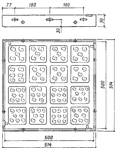
Рис. IV.1. Унифицированные ячейки фильтра Фя
