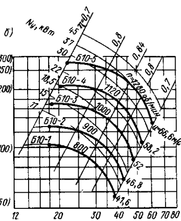
Рис. 1.11. Аэродинамические характеристики вентиляторов В.Ц4-75-10 (а), В.Ц4-75-12,5 (б), В.Ц4-75-16 (в) (исполнение б)
