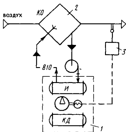
Рис 16.4. Одноконтурная схема присоединения воздухоохлаждающей машины к камере орошения 1 - водоохлаждающая машина, 2 - камера орошения, 3 - блок автоматического регулирования холодопроизводительности
