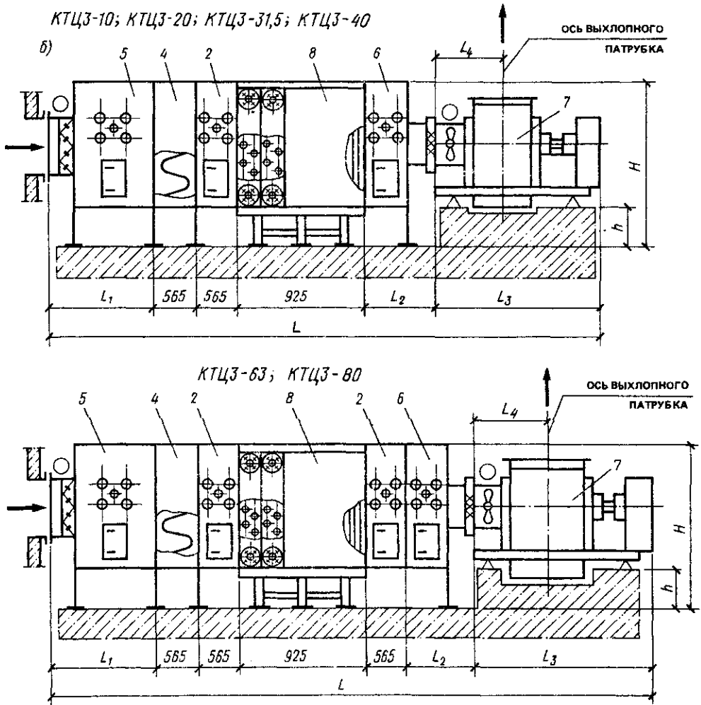
Рис. III.1. Центральные кондиционеры (базовые схемы 1, 2, 3) и кондиционеры-теплоутилизаторы (базовая схема 4) (б)
