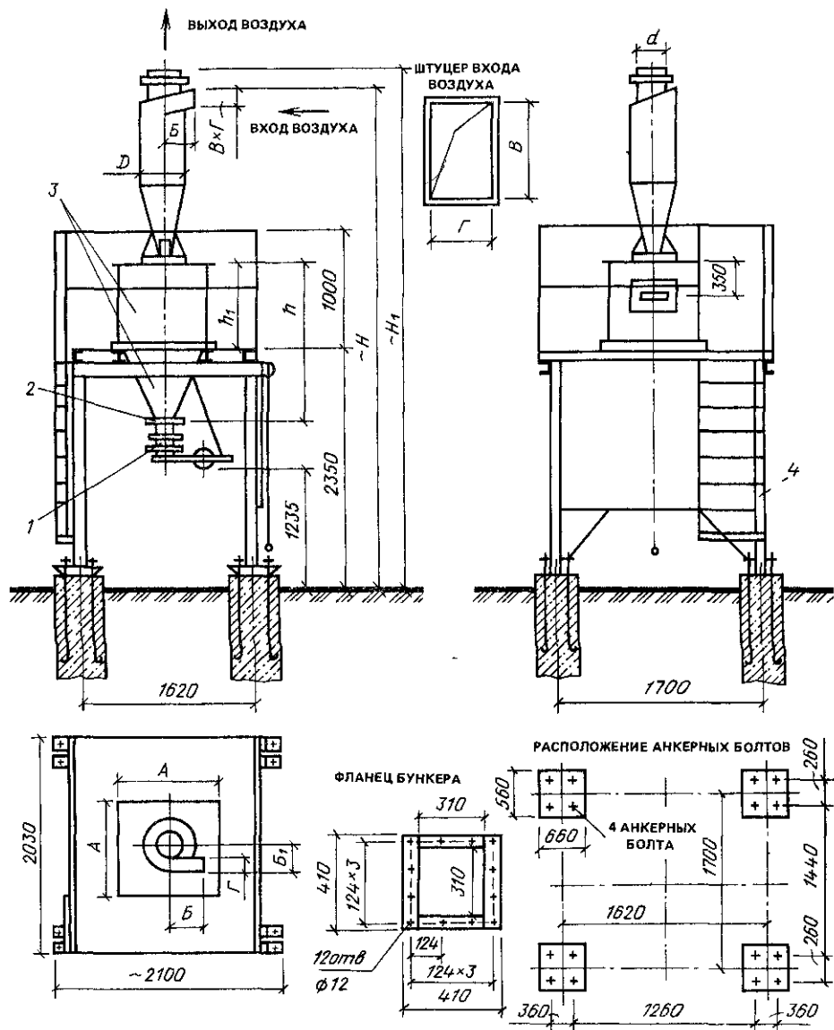
Рис. IV.9. Циклон ЦН-11 на постаменте
