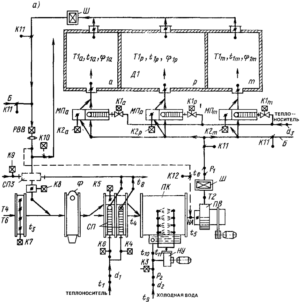
Рис. 15 11. Центральная многозональная двухвентиляторная система кондиционирования воздуха, работающая с рециркуляцией по одному или по двум каналам (второй канал показан пунктиром) а — схема системы, б — построение процессов на J - d -диаграмме при работе с одним первым рециркуляционным каналом, в — то же, при работе с двумя рециркуляционными каналами Примечание Воздухонагреватель СПЗ и клапан К9 устанавливаются в районах Крайнего Севера для предупреждения замерзания воздухоподогревателей первого подогрева
