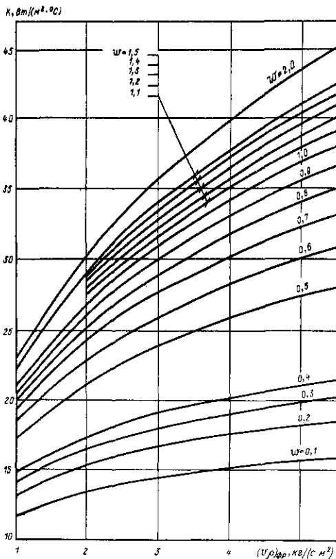
Рис. 21.6. Определение коэффициентов теплопередачи K воздухонагревателей КТЦ-3 двухрядных (раствор \text{CaCl}_2 ).
