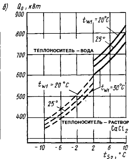
Рис. 16.2. Зависимости холодопроизводительности Q_0 от температуры хладонносителя t_{с2} и охлаждающей воды t_{w1} для хладоновой машины марки 21МКТ 280-2-1 (а) и 2МКТ 350-2-1 (б)
