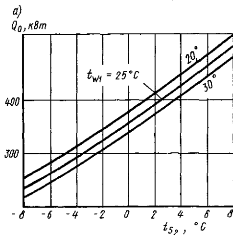
Рис. 16.2. Зависимости холодопроизводительности Q_0 от температуры хладонносителя t_{с2} и охлаждающей воды t_{w1} для хладоновой машины марки 21МКТ 280-2-1 (а) и 2МКТ 350-2-1 (б)
