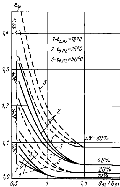
Рис. 21.9. Определение поправочных коэффициентов \xi_G и \xi_w
