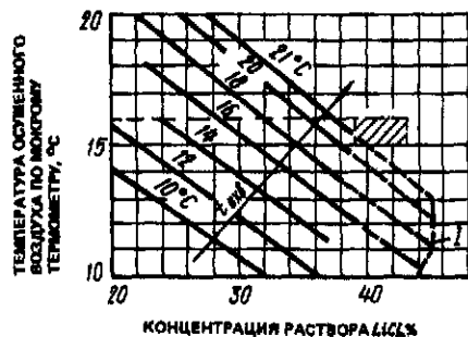
Рис. 15.53. Зависимость конечной температуры воздуха по мокрому термометру от концентрации водного раствора хлористого лития и температуры воды, охлаждающей раствор t_{\text{ср. в}} (по И. И. Чернобыльскому, О. А. Кремневу и А. С. Чавдарову)
