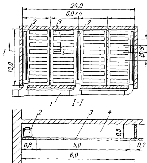
Рис. 18. Размещение перфорированных панелей на потолке (к примеру 42):
