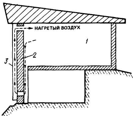
Рис. 16.3. Пассивная солнечная система отопления здания с естественной циркуляцией воздуха в пространстве между остеклением южного фасада и теплоаккумулирующей стеной 1 – здание; 2 – теплоаккумулирующая стена; 3 – остекление
