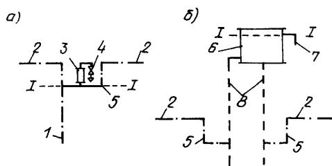
Рис. 10.16. Способы централизованного удаления воздушных скоплений из систем водяного отопления с нижней разводкой а — через вертикальный воздухоотборник; б — через расширительный бак; 1 — воздушная труба стояка; 2 — воздушные линии; 3 — вертикальный непроточный воздухоотборник; 4 — спускной кран; 5 — воздушная петля; 6 — открытый расширительный бак; 8 — соединительные трубы; 1–1 — верхний уровень воды
