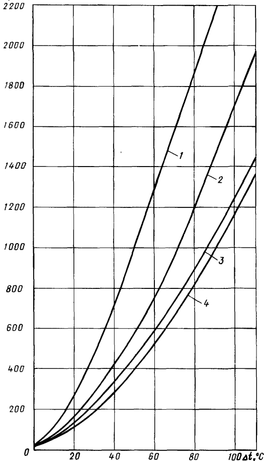
Рис. 13.17. График для определения теплоотдачи потолочных подвесных излучающих панелей q_{\text{пт}}
