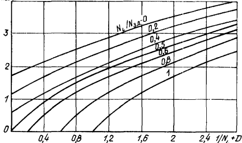
6.4. Зависимость B_{и.пом} от \left( \frac{1}{N_i} + D \right) и N_i / N_{зд}
