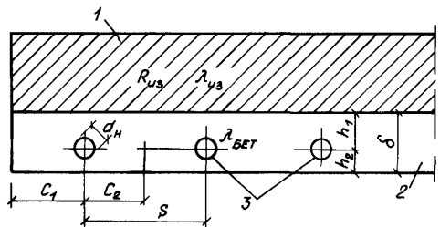
Рис. 13.14. Расчетная схема размещения нагревательных элементов в конструкции перекрытия (силовная плита)
