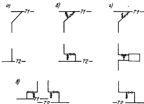
Рис. 10.13. Схемы присоединения стояков к магистралям систем отопления двух-трехэтажных зданий (а), четырех-семьэтажных при верхней разводке (б) и при нижней разводке (в), восьмиэтажных и более высоких зданий (г)
