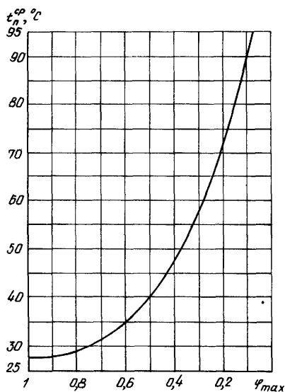
Рис. 13.18. Зависимость средней температуры поверхности панели от максимального коэффициента облученности человека панелями \varphi_{\max}
