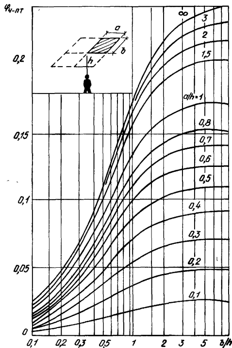
Рис. 13.19. Зависимость коэффициента облученности человека с поверхности потолка \varphi_{\text{ч-пт}} от геометрии помещения
