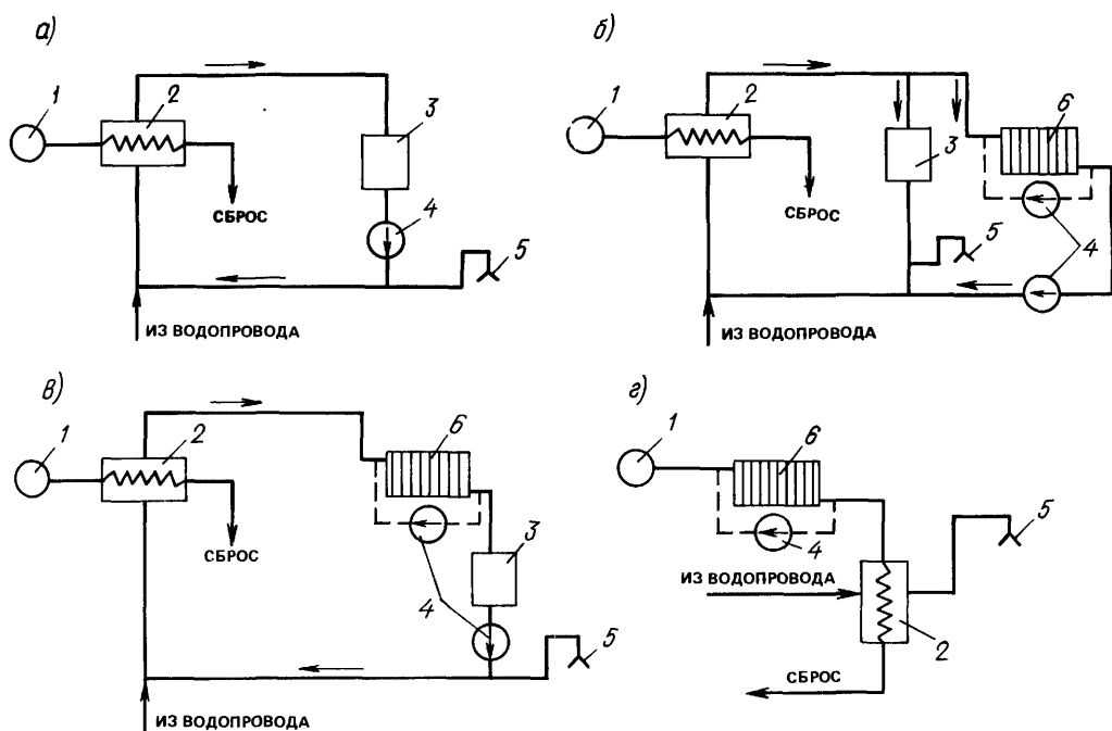
Рис. 17.11. Схемы двухконтурных (а, б) и комбинированной (з) систем геотермального теплоснабжения
