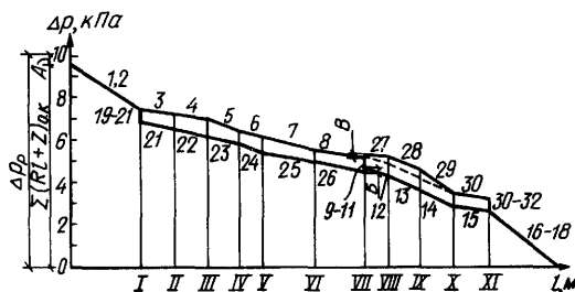
Рис. 10.23. Эпюра циркуляционного давления в двухтрубной системе отопления с попутным движением воды в магистралях (см. рис. 10.22)
