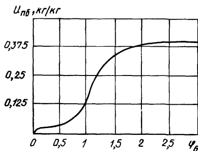
Рис. 4.2. Зависимость равновесного влагосодержания пенобетона U_{пб} от относительного потенциала влажности \varphi_{\theta}
