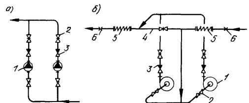
Рис. 10.2. Схемы присоединения труб к циркуляционным бесфундаментным (а) и общепромышленным (б) насосам
