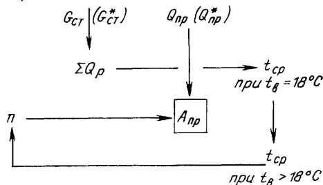
Рис. 9.2. Ключ к табл. 9.8 для определения требуемой площади A_{пр} отопительных приборов при t_n = 18^\circ\text{C} (а), при t_n < 18^\circ\text{C} (б), при t_n > 18^\circ\text{C} (в)
