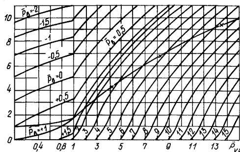
6.1. Зависимость B_{и.пом} от \bar{p}_{вн} и (\bar{p}_{вн}, \bar{p}_a)
