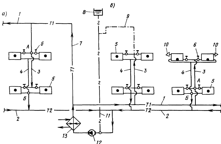
Рис. 10.9. Схема вертикальной двухтрубной системы насосного водяного отопления с верхней разводкой (а), с нижней разводкой (б) 1 и 2—подающие и обратные магистрали; 3 и 4—подающие и обратные стояки; 5—отопительные приборы; 6—краны двойной регулировки; 7—главный стояк; 8—расширительный бак; 9—воздушная линия; 10—воздушные краны; 11—соединительная труба расширительного бака; 12—циркуляционный насос; 13—теплообменник
