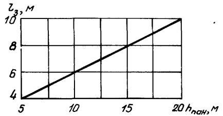
Рис. 13.8. Зависимость расстояния от крайних подвесных излучающих панелей до стен l_3 от высоты их подвеса h_{\text{пан}}
