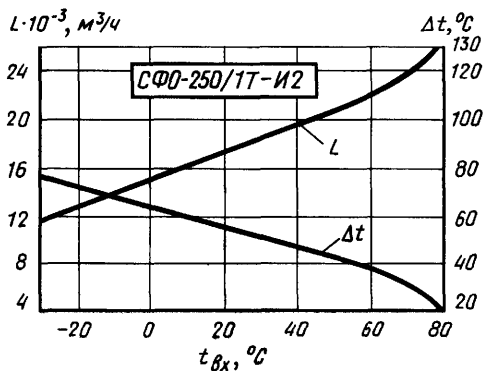
Рис. 14.1. Зависимости минимально допустимой производительности по воздуху L и перепада температур выходящего и входящего воздуха \Delta t от температуры входящего воздуха (при температуре выходящего воздуха до 50^\circ\text{C} )
