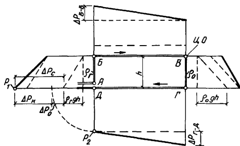
Рис. 10.11. Эшюра гидравлического давления в системе отопления, непосредственно соединенной с наружными теплопроводами В-точка наименьшего давления, Г-точка наибольшего давления, Д-точка постоянного давления в системе
