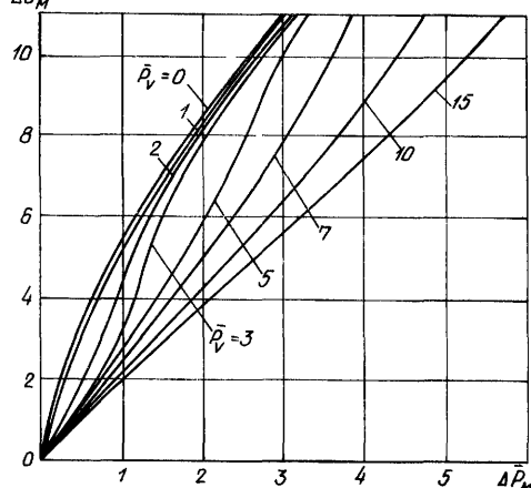
6.2. Зависимость \Delta \bar{p}_м от \Delta \bar{G}_м и \bar{p}_v
