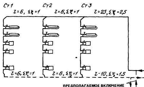
Рис. 10.27. Схема одноконтурной системы водяного отопления со стояками унифицированной конструкции и тупиковым движением воды в магистралях (к примеру 10.12)
