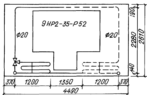
Рис. 13.3. Стеновая совмещенная панель конструкции Челябинскогогражданпроекта
