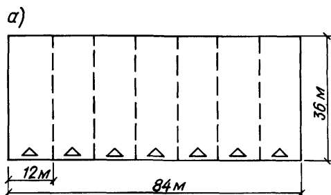
Рис. 12.2. План производственного цеха. Схема наклонной подачи воздуха агрегатами А02-6,3 О1У3
