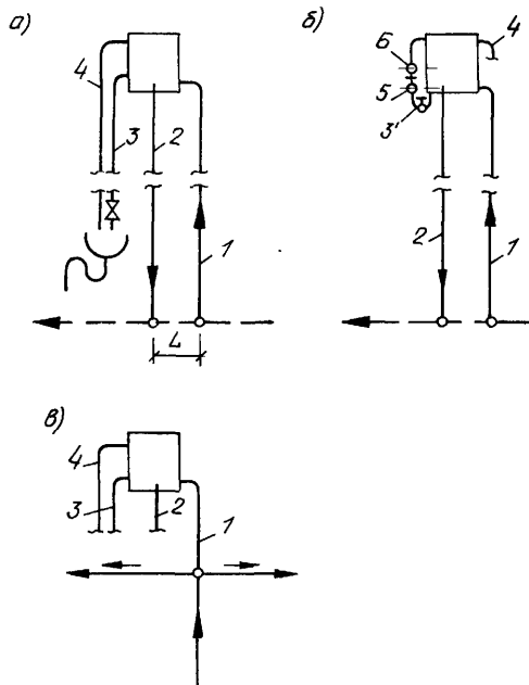
Рис. 10.18. Присоединение открытого расширительного бака к магистралям
