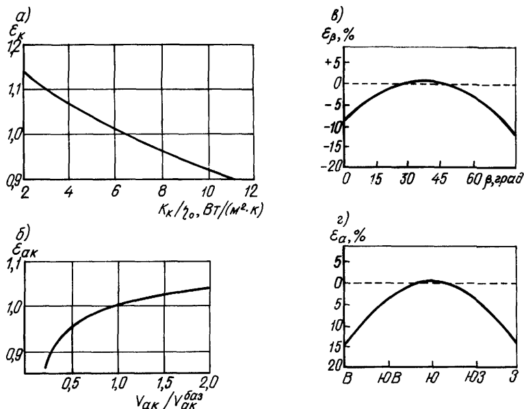
Рис. 16.20 Графики для определения поправочных коэффициентов \epsilon_k , \epsilon_{ак} , \epsilon_\beta , \epsilon_a
