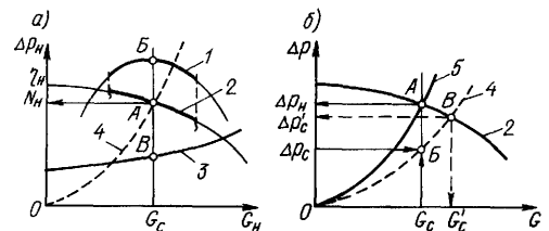
Рис. 10.3. Характеристики циркуляционных насосов
