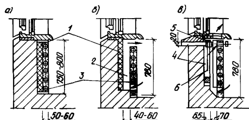
Рис. 13.4. Подоконные приставные бетонные панели
