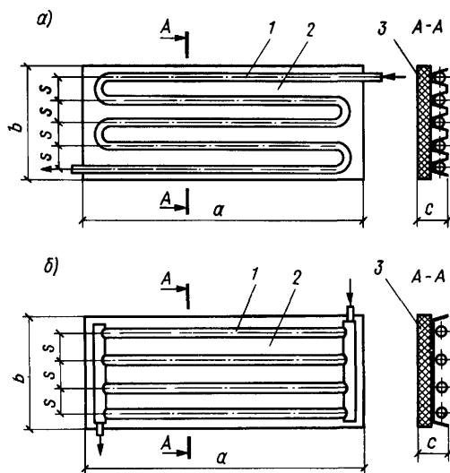
Рис. 13.6. Подвесные излучающие панели с гофрированным (а) и плоским экраном (б)
