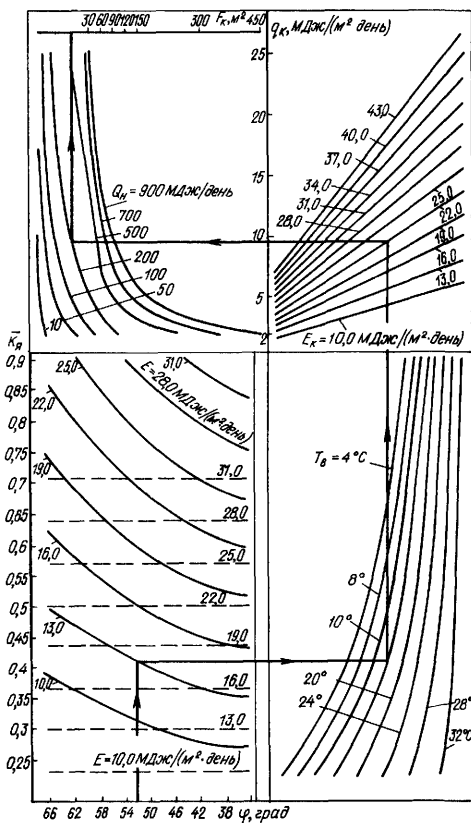
Рис. 16.18. Номограмма для определения среднесуточного поступления солнечной энергии E_d на поверхность КСЭ с оптимальным углом наклона и ориентацией
