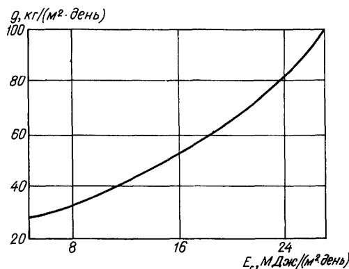
Рис. 16.17. Зависимость удельной суточной производительности систем солнечного горячего водоснабжения от суммарного поступления солнечной энергии E_{г.} на горизонтальную поверхность
