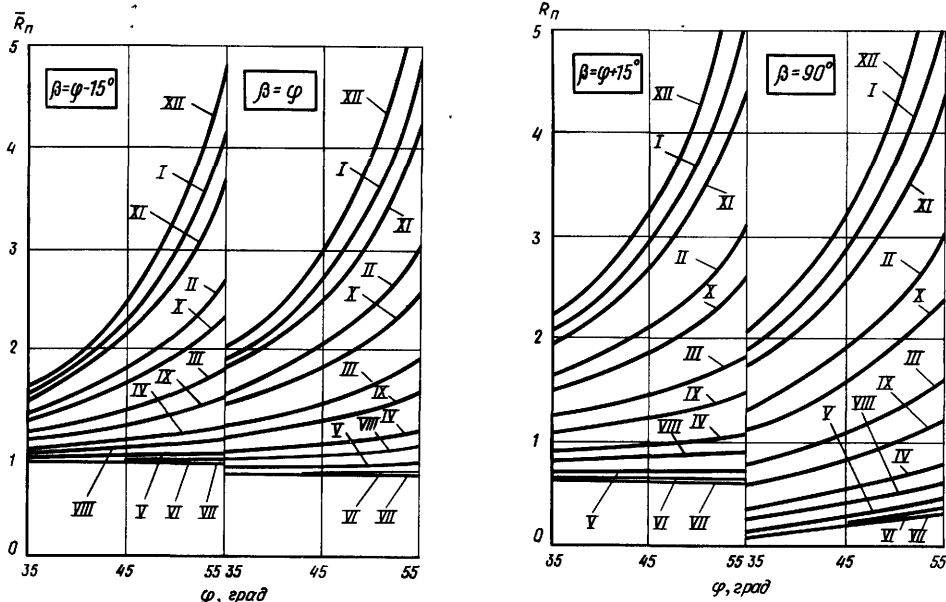
Рис. 16.8. Зависимость среднемесячного коэффициента пересчета прямого солнечного излучения \bar{R}_n с горизонтальной плоскости на поверхность КСЭ от широты местности \varphi для I–XII месяцев года
