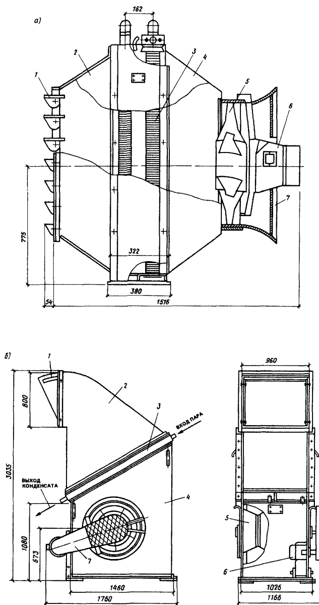
Рис. XI.2. Воздушно-отопительные агрегаты STD-300П (а) и STD-300M-01.Y3 (б)
