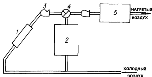
Рис. 16.4. Принципиальная схема воздушной гелиосистемы отопления
