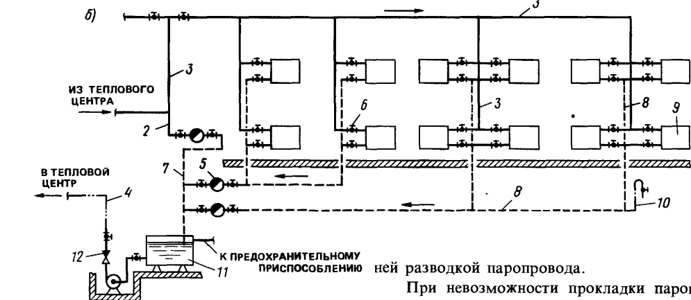
Рис. 11.3. Схемы закрытых систем парового отопления высокого давления замкнутой (а) и разомкнутой (б)
