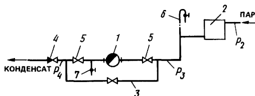
Рис. 11.14. Схема установки конденсатоотводчика
