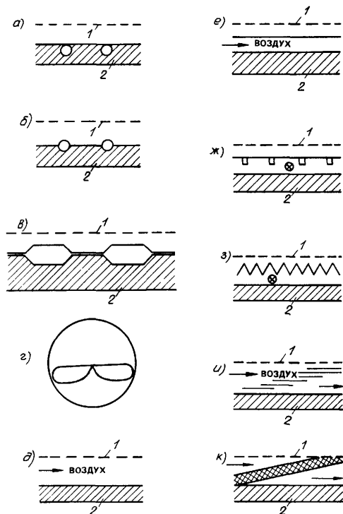
Рис. 16.10. Схемы жидкостных (а-г) и воздушных (д-к) коллекторов солнечной энергии
