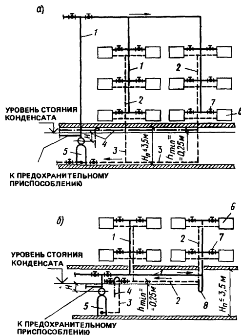
Рис. 11.1. Схемы систем парового отопления низкого давления замкнутых открытых
