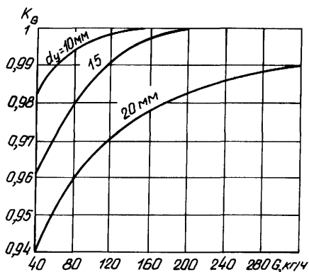
Рис. 13.11. Зависимость поправочного коэффициента K_G от расхода воды G при различных диаметрах труб нагревательных элементов
