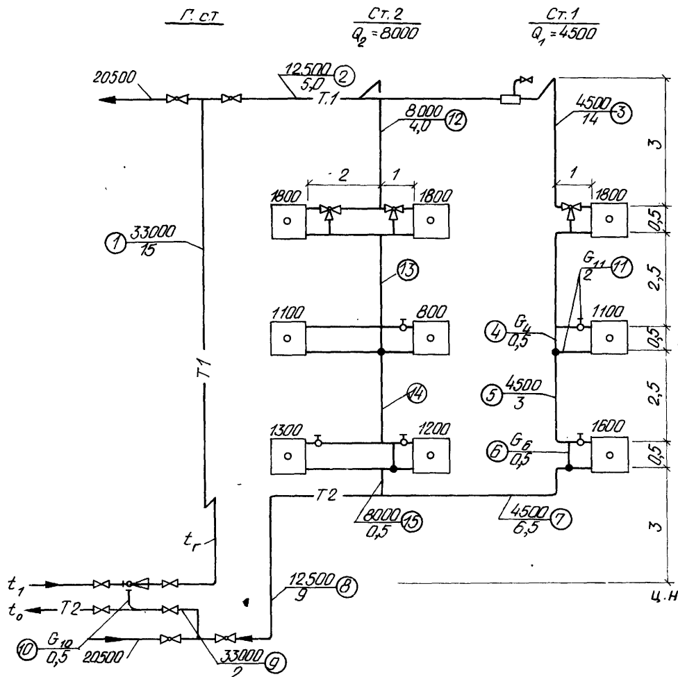
Рис. 10.21. Схема вертикальной однотрубной системы водяного отопления с верхней разводкой и тупиковым движением воды в магистралях (к примеру 10.1)
