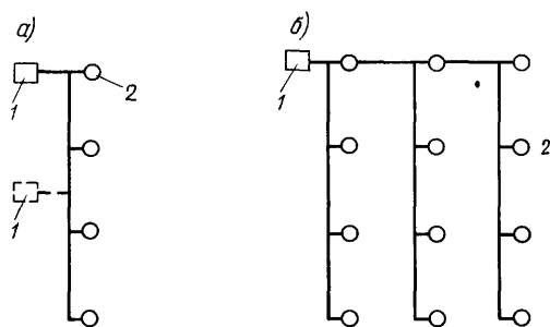
Рис. 17.12. Варианты объединения скважин
