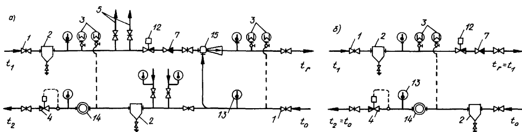
Рис. 10.6. Принципиальные схемы местного теплового пункта при непосредственном присоединении системы водяного отопления к наружным теплопроводам со смещением воды с помощью водоструйного элеватора 15 (а) и без смещения воды (б)
