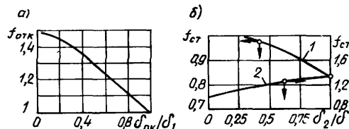
Рис. 2.4. Значение фактора формы откоса проема (а) и стыка наружной стены и внутренней перегородки (б) по наружному обмеру (1) и по внутреннему (2)
