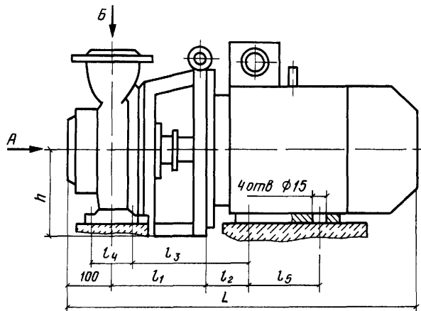
ВИД А
