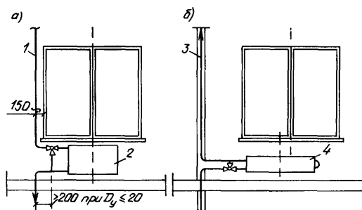
Рис. 10.12. Узлы вертикальных проточно-регулируемых одноконтурных систем отопления с присоединяемыми стояками и радиаторами (вертикальные оси приборов в окнах совпадают) (а), с замоноличенными в перегородки стояками и конвекторами (приборы смещены к стоякам от вертикальной оси окон) (б) 1—прикоконный стояк, 2—радиатор, 3—замоноличенный стояк, 4—конвектор
