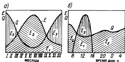
Рис. 16.15. Типичные годовой (а) и суточный (б) графики изменения количества поступающей солнечной энергии E и тепловой нагрузки теплоснабжения здания Q
