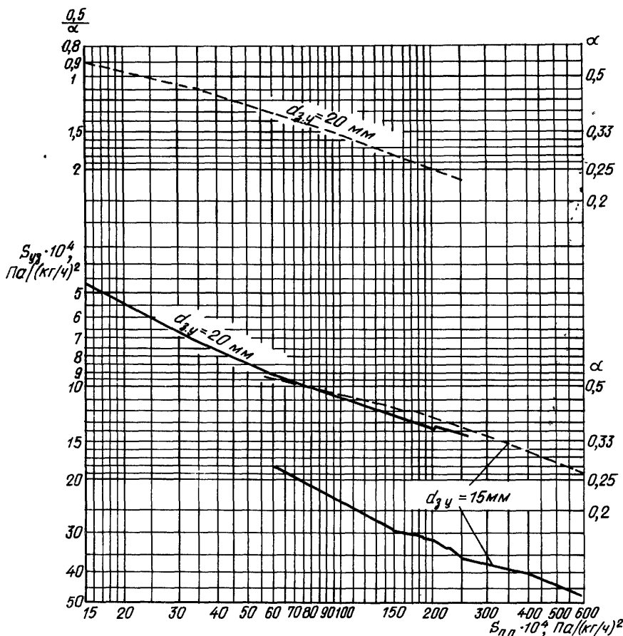
Рис. 10.25. Зависимость характеристик сопротивления S_{yz} \cdot 10^4 (сплошные линии) и коэффициента затекания \alpha (пунктирные линии) приборного узла со смещенным замыкающим участком в вертикальной однотрубной системе отопления от характеристик сопротивления подводки с прибором S_{nn} \cdot 10^4 ( d_{zy} - диаметр замыкающего участка)
