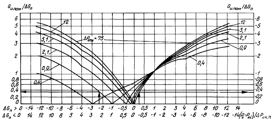
6.5. Зависимость G_{n, \text{пом}}/\Delta G_n от отношения p_0 - p_{n_i}/\Delta p_{\text{ок}, \text{п}}
